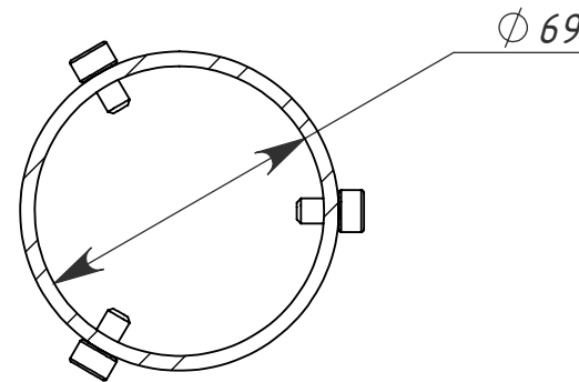
СЕЧЕНИЕ В-В МАСШТАБ 1:2
